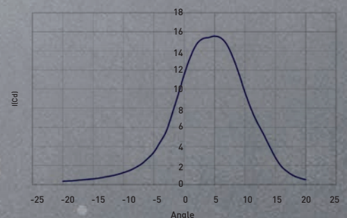
Representación cartesiana de la distribución angular de intensidad luminosa (10 Cd.) en los semiplanos verticales.
